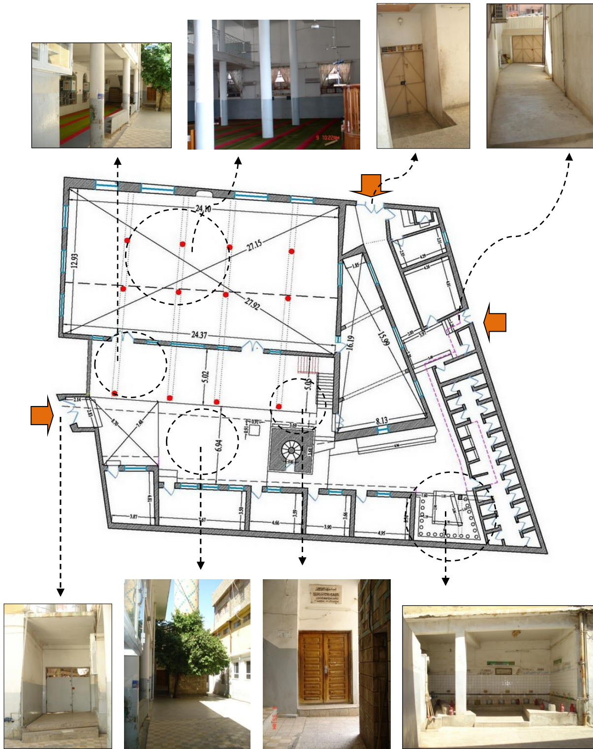
شكل رقم (3 أ) : عملية التوثيق للجامع الكبير بمدينة دهوك (واقع الحال) ، مخطط الطابق الارضي ، (إعداد : الباحثة) .
